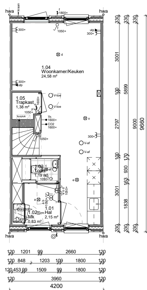
Begane grond
