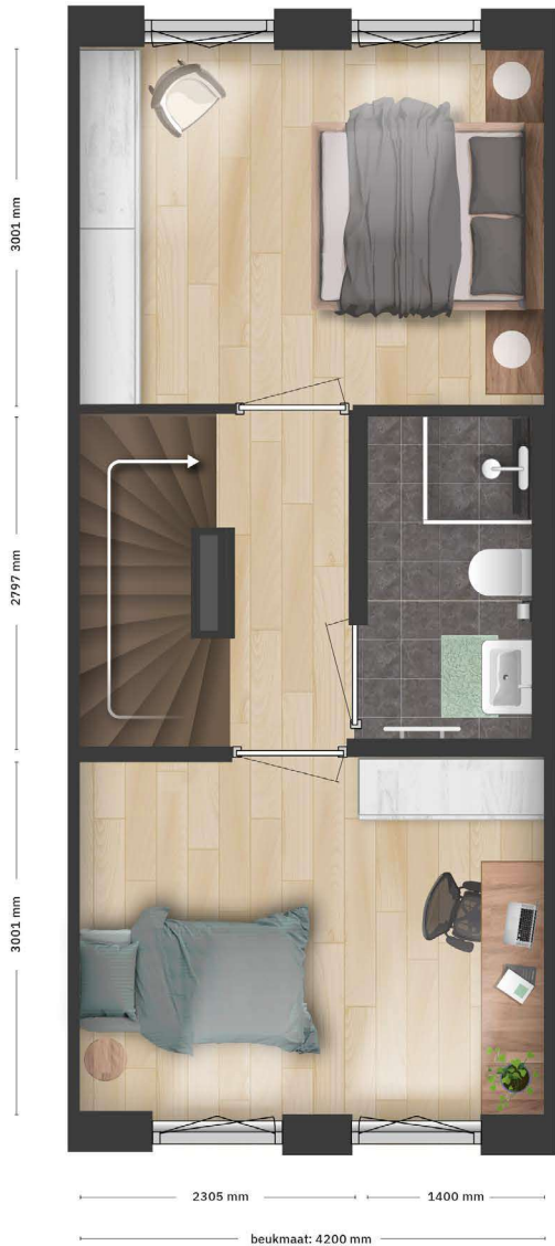
Eerste verdieping
